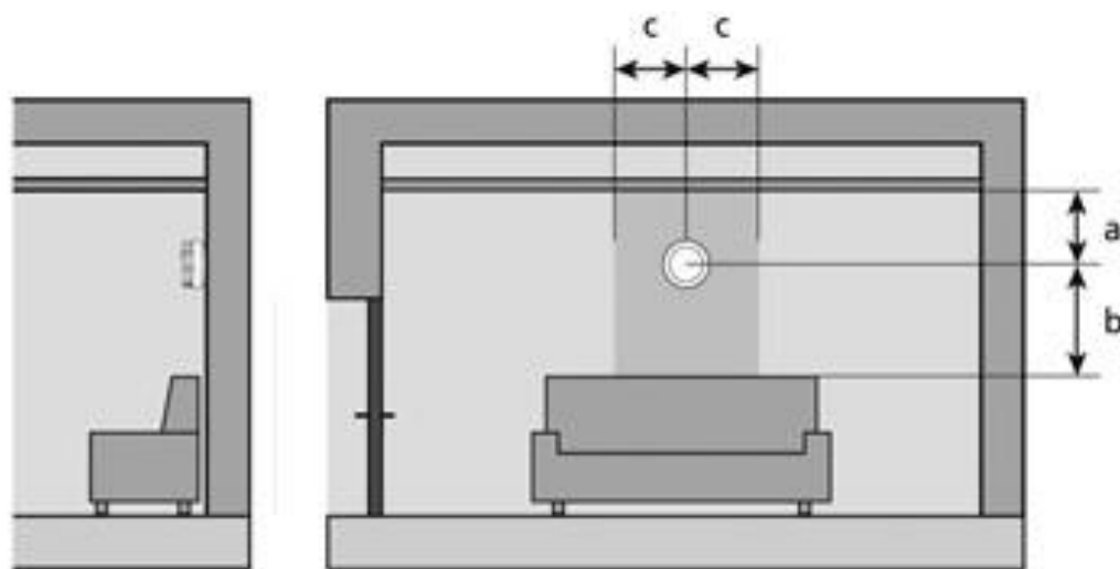
Vægmontering af en røgalarm
